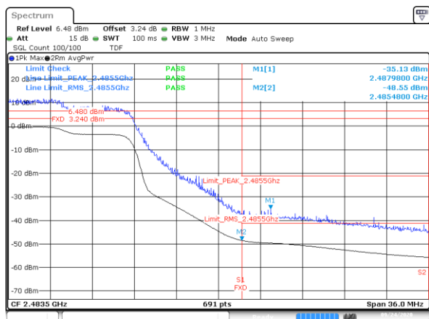
BE-R-HIGH, MIMO-A, 802.11ax40-HE0, Ch12
