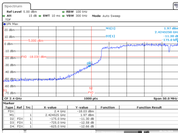
BE-NR, MIMO-A, 802.11ax40-HE0, Ch1
