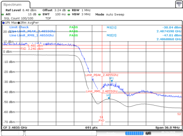
BE-R-HIGH, MIMO-A, 802.11ax40-HE0, Ch13
