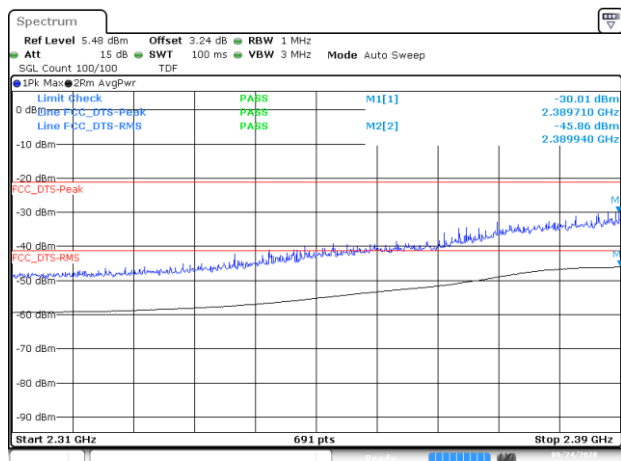
BE-R-LOW, MIMO-A, 802.11ax40-HE0, Ch1
