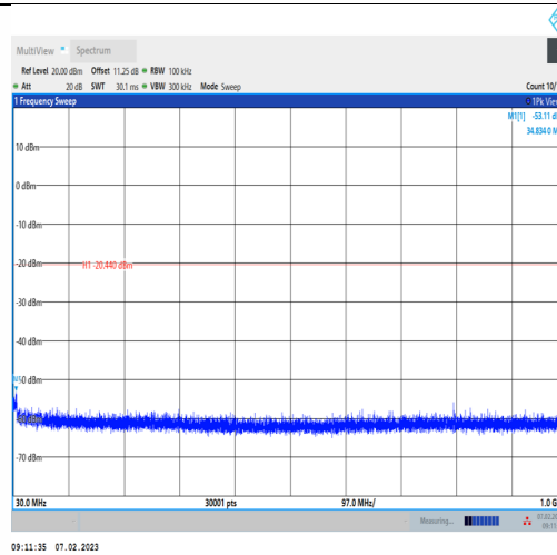
2DH5-Ant1-2402-30~1000--0.44
