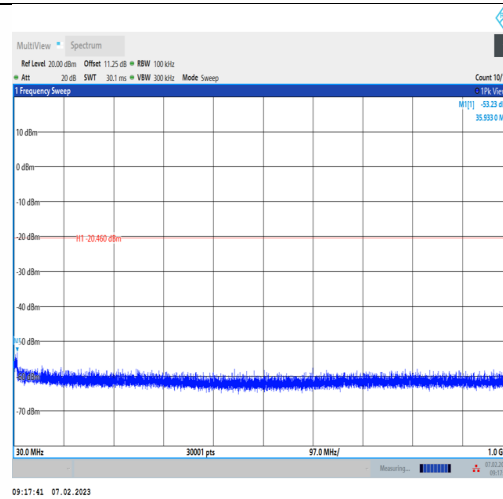
3DH5-Ant1-2402-30~1000--0.46
