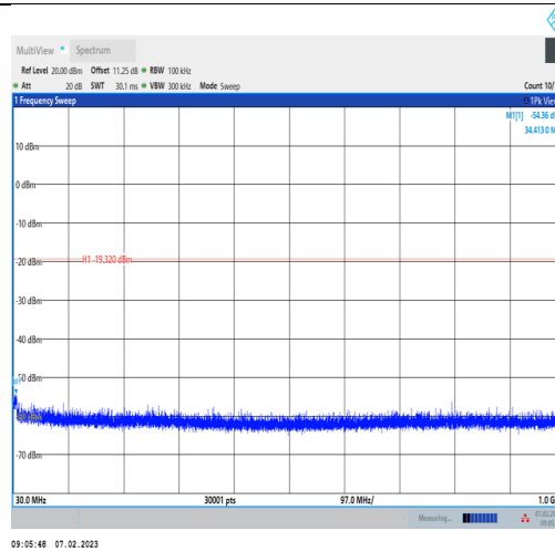
DH5-Ant1-2402-30~1000-0.68
