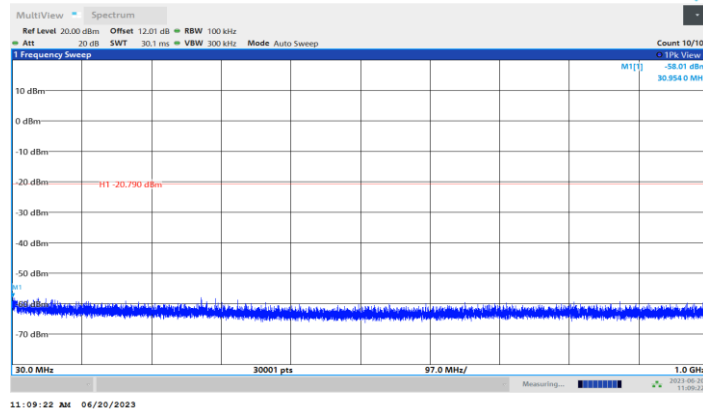
BLE_2M_Ant1_2480_30~1000
