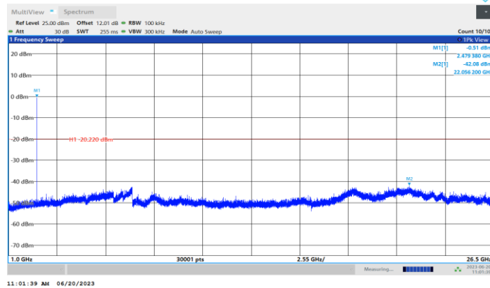
BLE_1M_Ant1_2480_1000~26500
