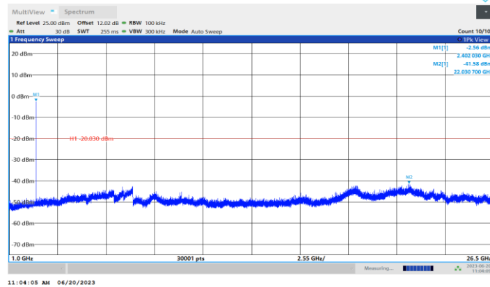
BLE_2M_Ant1_2402_1000~26500
