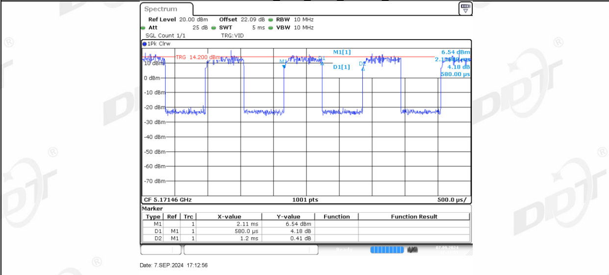
11AX20MIMO_Ant1_5180_26Tone_RU4
