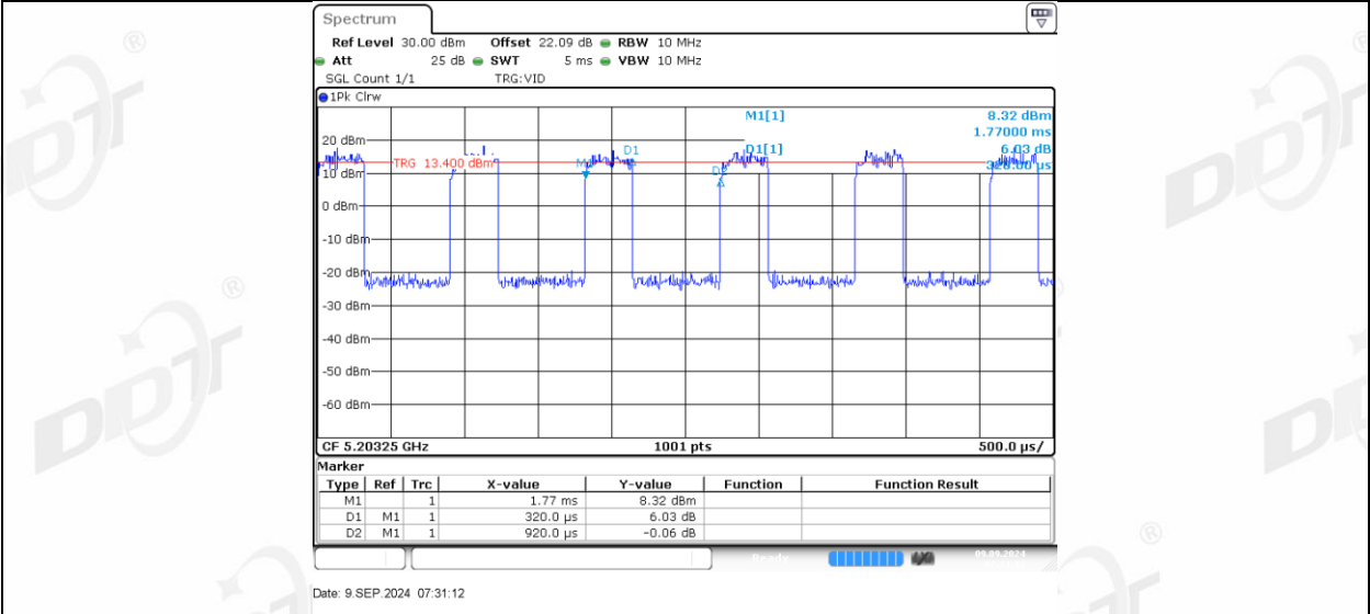
11AX20MIMO Ant1 5200 52Tone RU40
