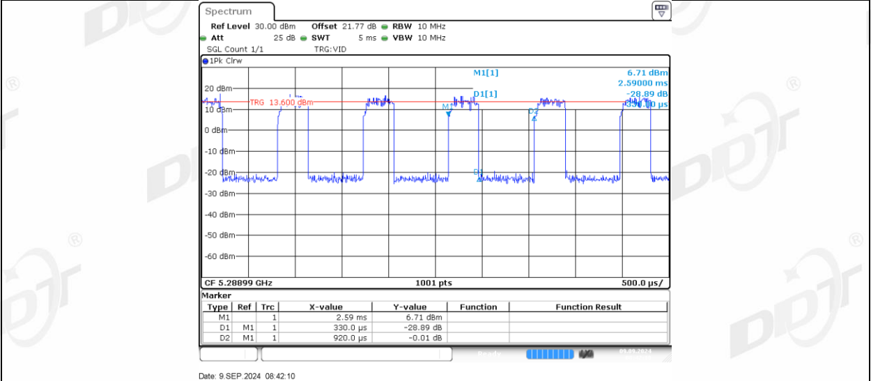
11AX20MIMO Ant1 5280 106Tone RU53
