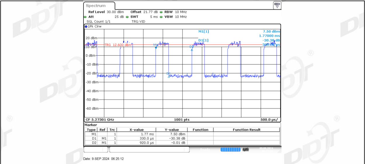
11AX20MIMO Ant1 5280 52Tone RU39
