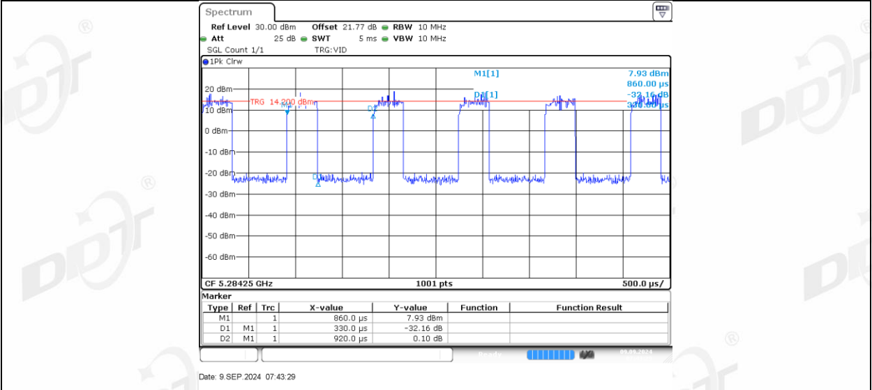
11AX20MIMO Ant1 5280 52Tone RU40
