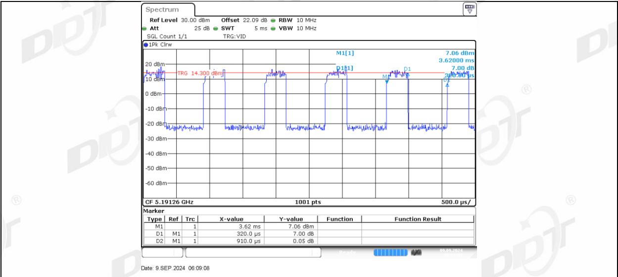
11AX20MIMO Ant1 5200 52Tone RU39
