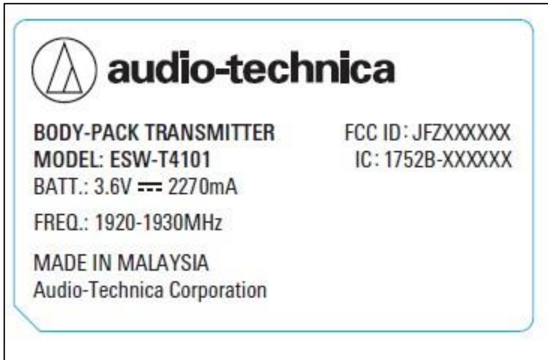
Photo 5: DUT - Label
