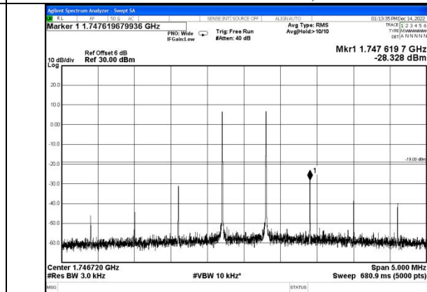
AWS Band AGC+10dB, UL
