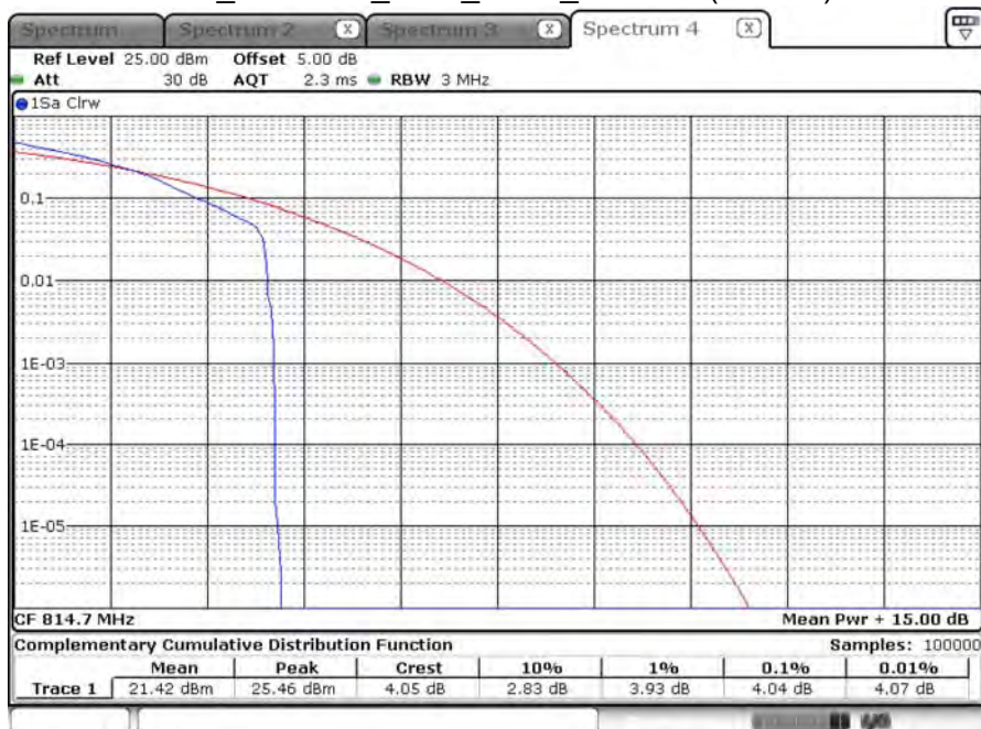
B26_CH26697_1.4M_1RB2_16-QAM (Part 90)
