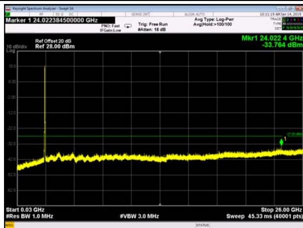
FDD7_MiddleRange_15+10MHz_30MHz~26GHz
