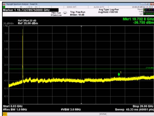
FDD7_HighRange_20+10MHz_30MHz~26GHz
