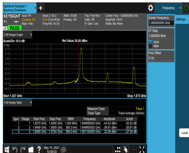
Band2-20MHz-16QAM-18700-100RB#0
