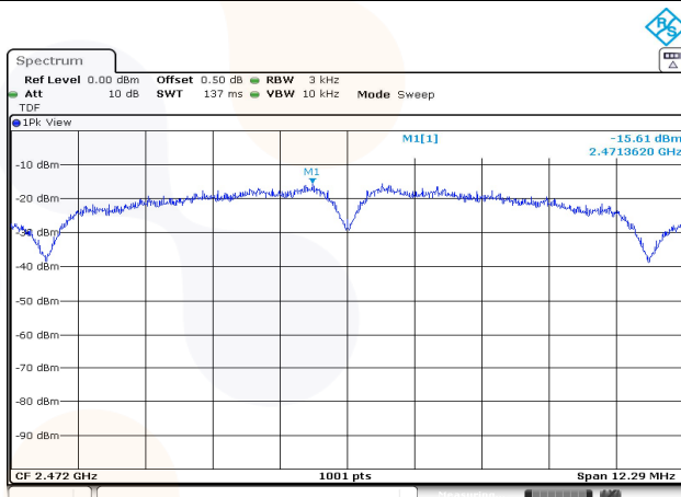
802.11b / 2 472 MHz
