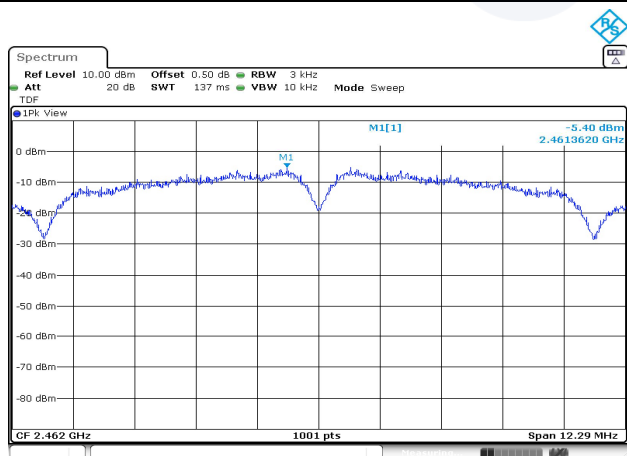
802.11b / 2 462 MHz
