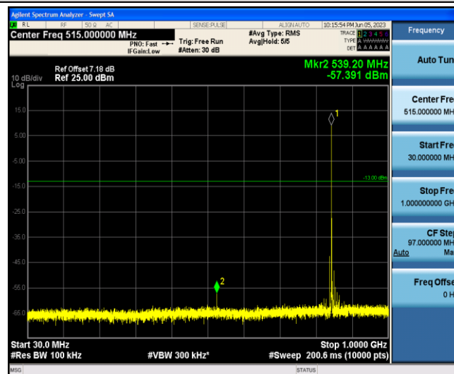
Band5-3MHz-QPSK-20635-1-0-Low-30-1000--57.39-PASS
