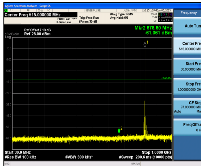
Band5-3MHz-QPSK-20525-1-0-Low-30-1000--61.06-PASS
