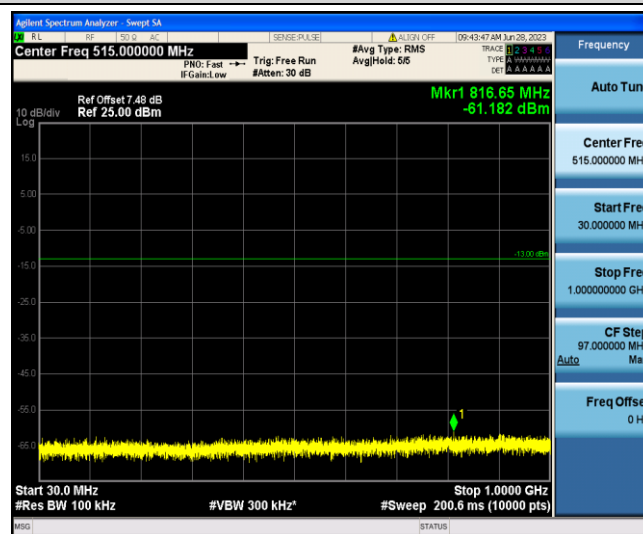
Band4-10MHz-QPSK-20350-1-0-Low-30-1000--61.18-PASS
