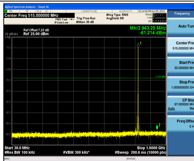
Band5-3MHz-16QAM-20415-1-0-Low-30-1000--61.21-PASS
