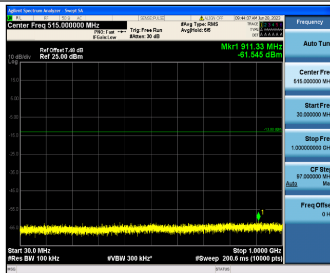
Band4-10MHz-16QAM-20350-1-0-Low-30-1000--61.55-PASS
