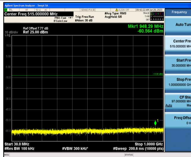
Band4-10MHz-QPSK-20000-1-0-Low-30-1000--60.56-PASS
