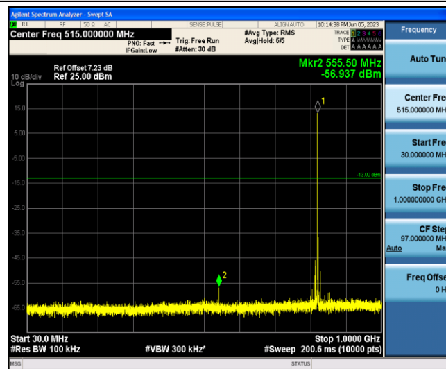
Band5-3MHz-QPSK-20415-1-0-Low-30-1000--56.94-PASS
