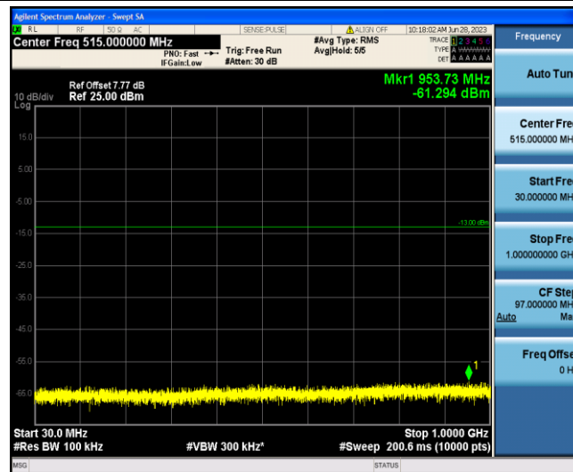
Band4-20MHz-QPSK-20050-1-0-Low-30-1000--61.29-PASS
