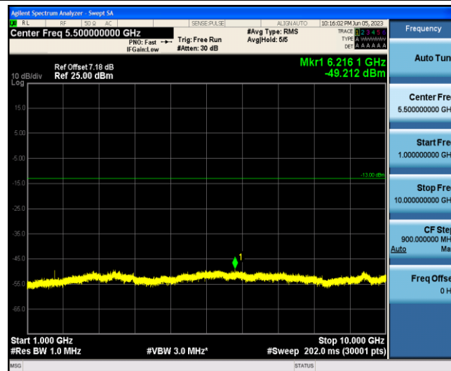
Band5-3MHz-QPSK-20635-1-0-Low-1000-10000--49.21-PASS
