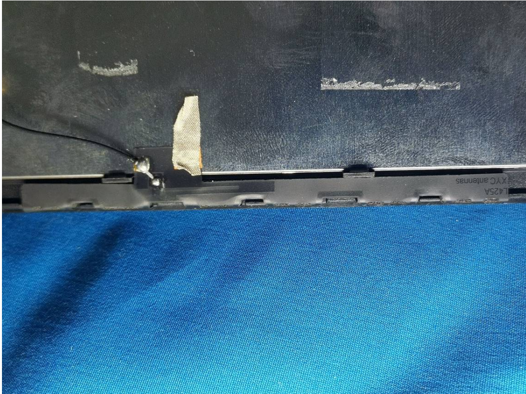
GSM/WCDMA Antenna
