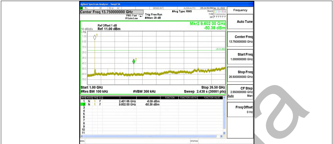
DH5_Ant1_2402_1000~26500
