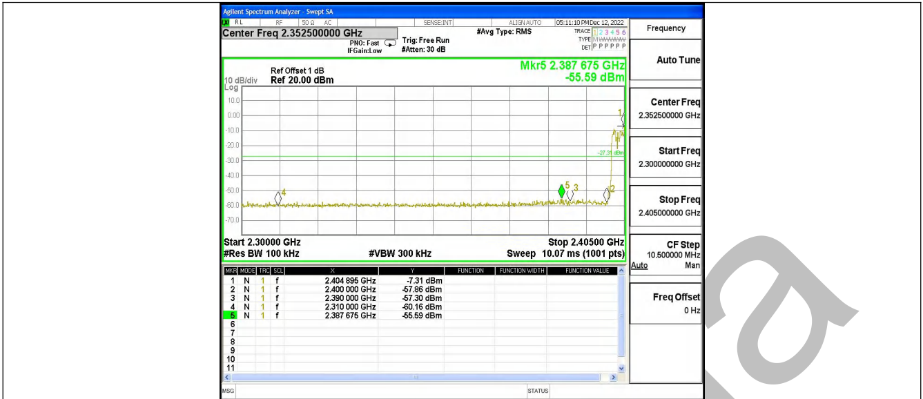
3DH5_Ant1_Low_Hop_2402
