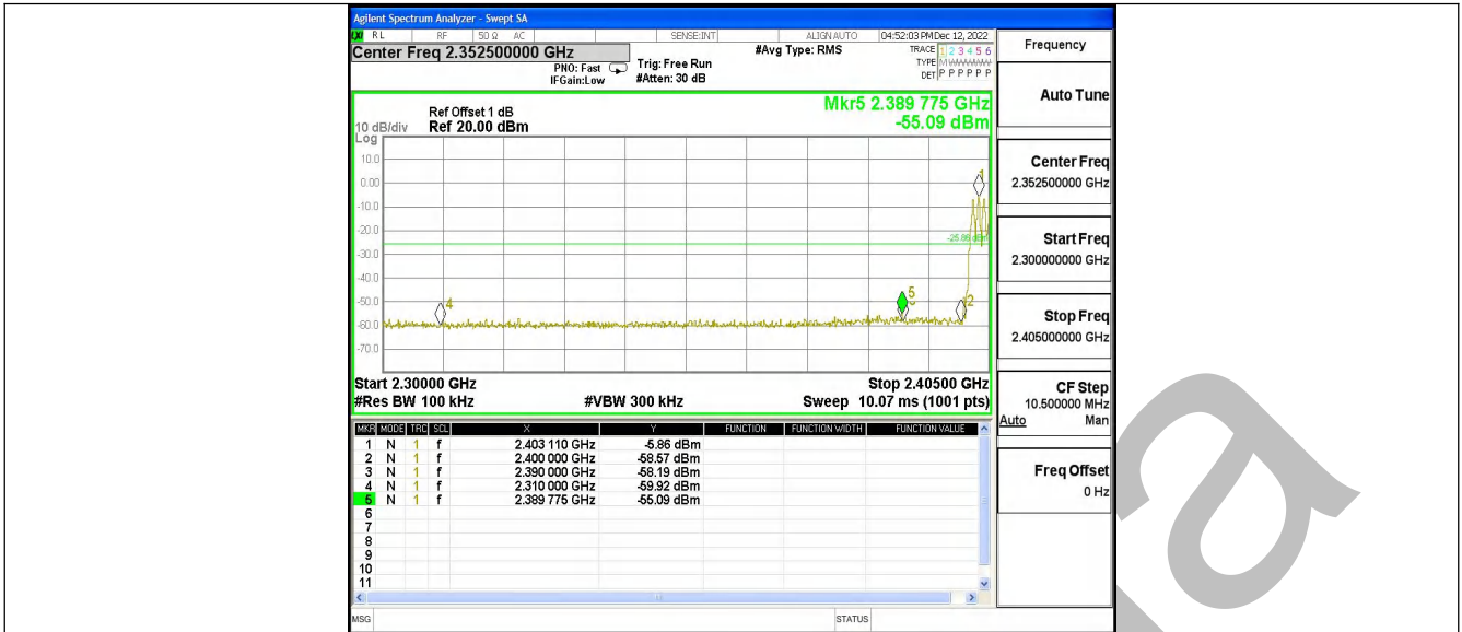
DH5_Ant1_Low_Hop_2402
