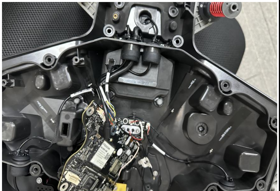
Antenna
