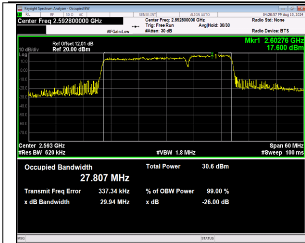
41-41-20MHz-10MHz-QPSK-QPSK-40571-40715-100RB#0-50RB#0-PASS
