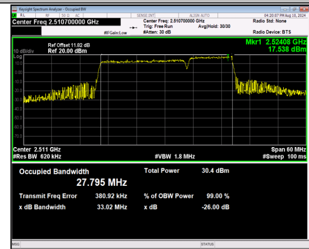
41-41-20MHz-10MHz-QPSK-QPSK-39750-39894-100RB#0-50RB#0-PASS
