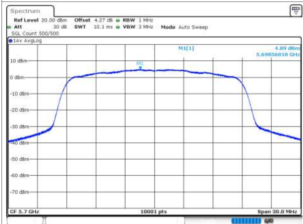
PSD NVNT n20 5700MHz Ant1
