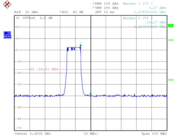
2472.5 MHz
