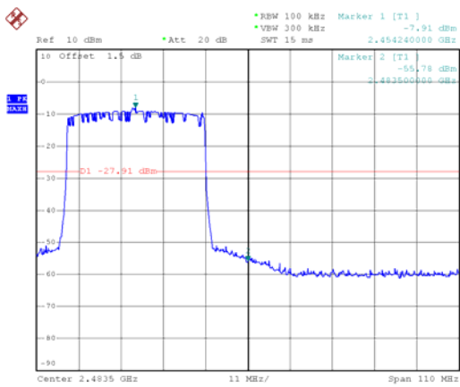
2454.5 MHz
