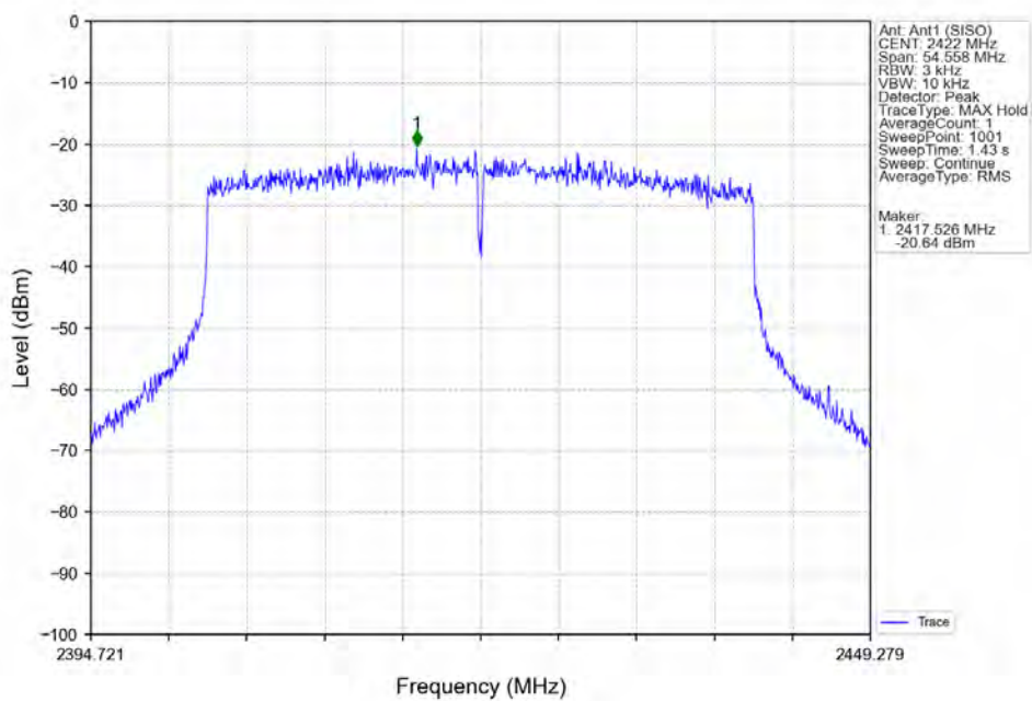
802.11ax(HE40)_LCH_2422MHz_RU484_Left_Ant1 (SISO)_NTNV
