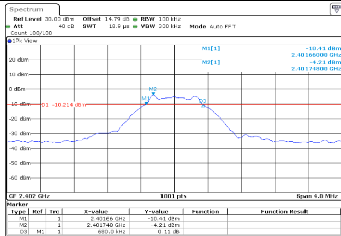
BLE_Ant1_2402
