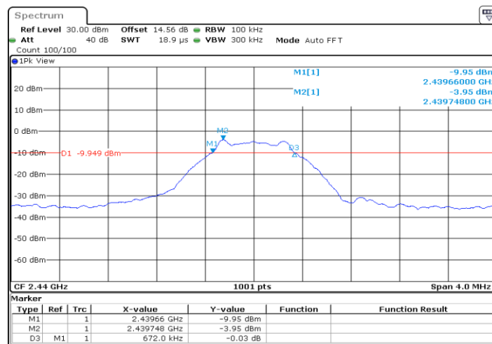
BLE_Ant1_2440
