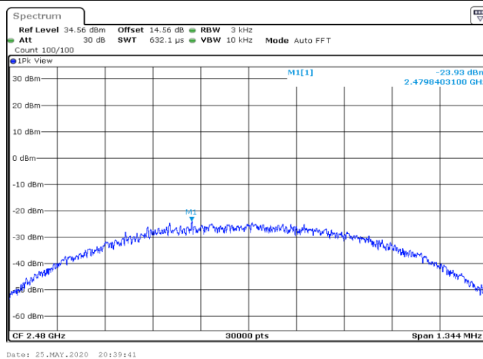
BLE_Ant1_2480
