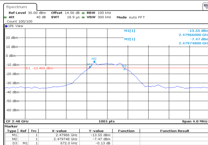
BLE_Ant1_2480
