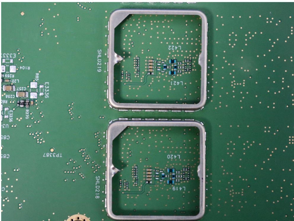
(41) EUT Photo
