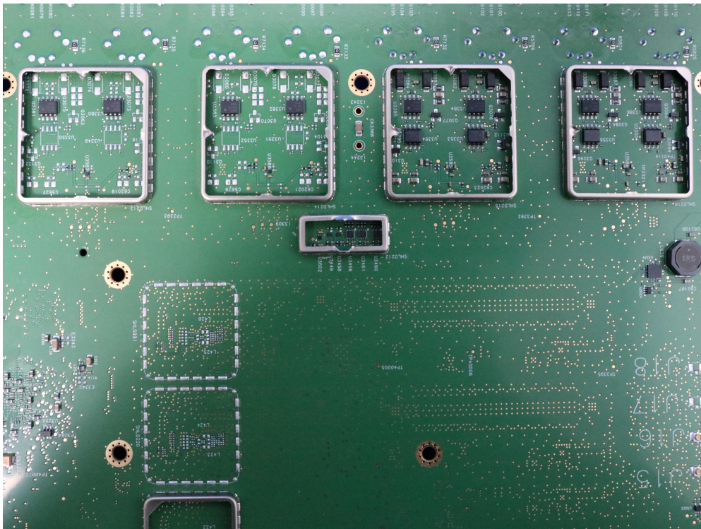
(40) EUT Photo
