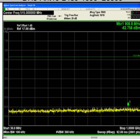
2DH5-Ant10-2402-30~1000
