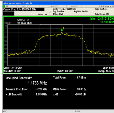
3DH5-Ant10-2441
