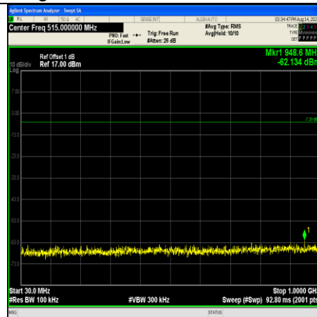
DH5-Ant10-2480-30~1000
