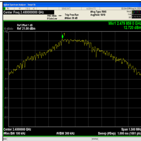
DH5-Ant10-2480-0~Reference
