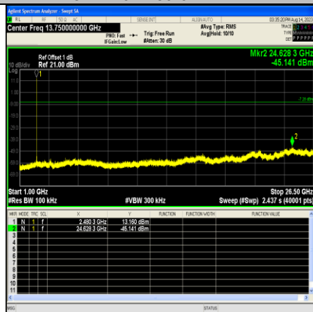
DH5-Ant10-2480-1000~26500
