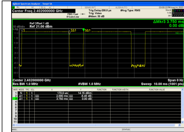
NTNV-DH5-Ant10-2402
