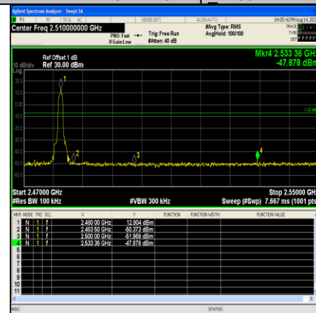
3DH5-Ant10-2480
