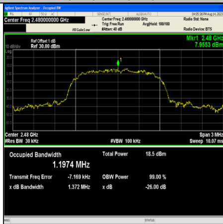
3DH5-Ant10-2480
