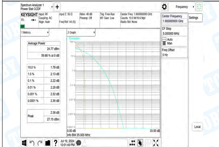
Band2-20MHz-16QAM-18700-1RB#0-PASS
