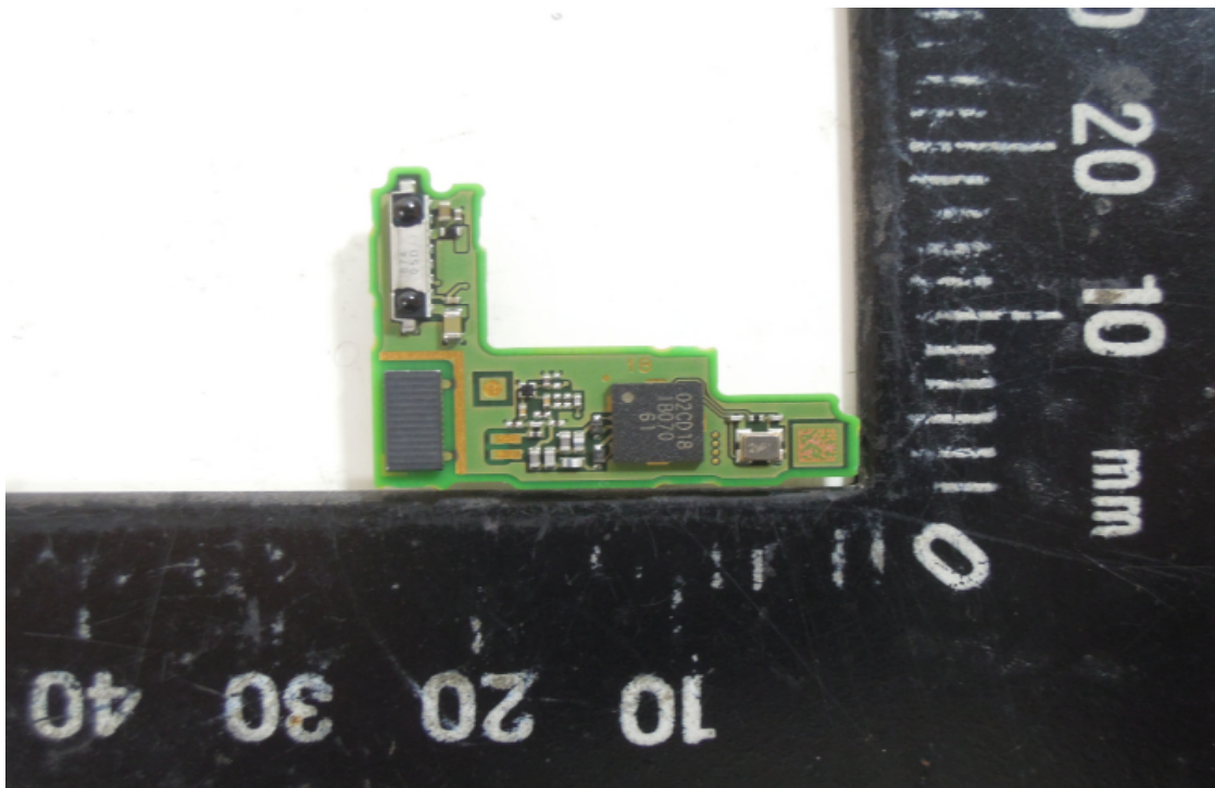
BT / WLAN / WWAN (Aux) / WWAN (Main) Antenna
