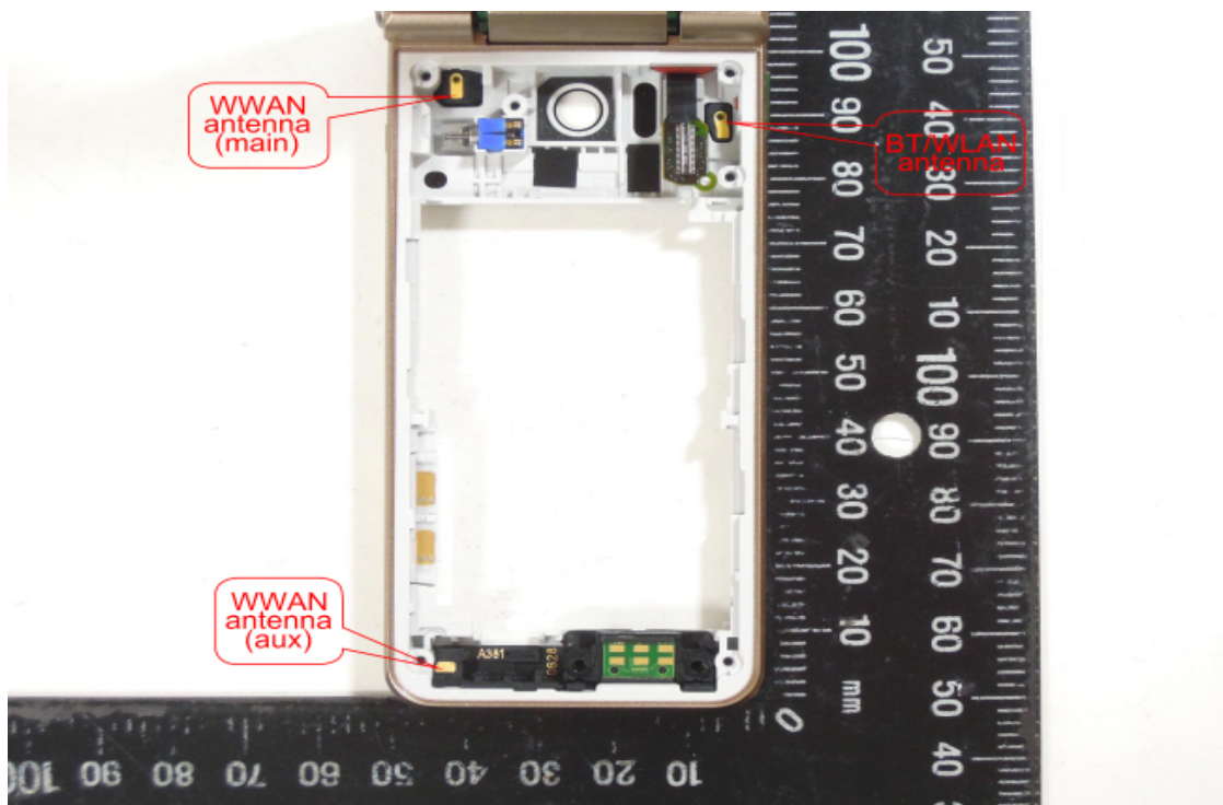
BT / WLAN / WWAN (Aux) / WWAN (Main) Antenna
