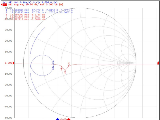
S Parameter (Return Loss, Smith)
