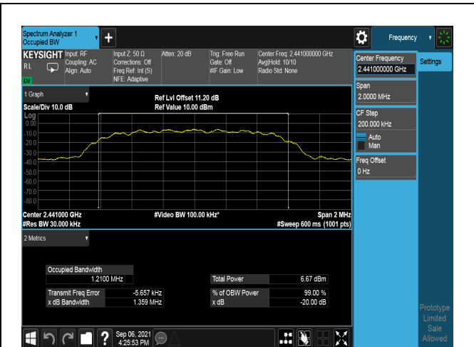
Modulation: \pi/4 DQPSK 2441MHz
