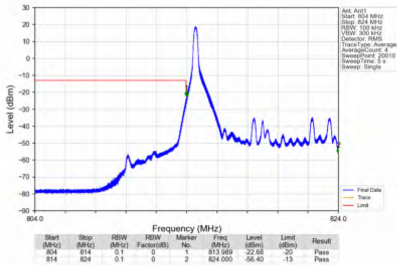
Band26a_10MHz_QPSK_LCH_819MHz_RB_1_0_NTNV
