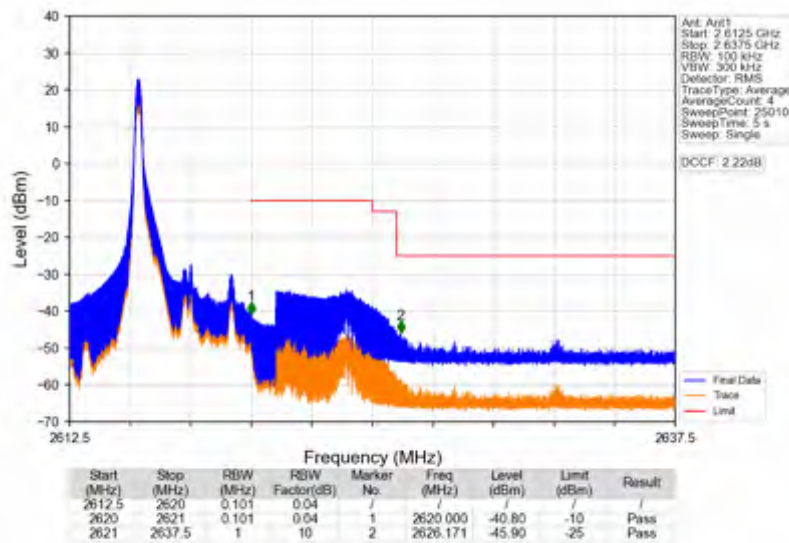
Band38_5MHz_QPSK_HCH_2617.5MHz_RB_1_24_NTNV
