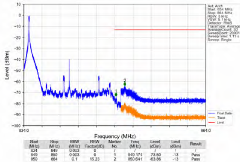
Band26c_15MHz_16QAM_HCH_841.5MHz_RB_1_74_NTNV
