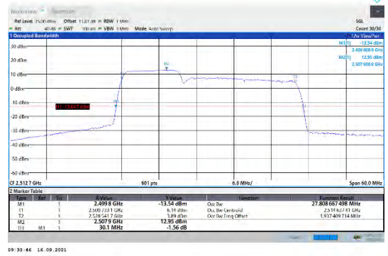
CA_7C-10MHz-20MHz-QPSK-QPSK-20805-20949-50RB#0-100RB#0
