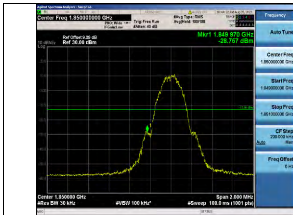
EGPRS1900-512
