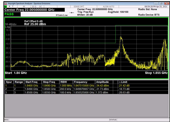
N2(20M)_DFT-s-OFDM_QPSK_Edge_1RB_Lef t_Low_CH
