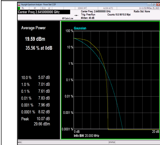
41(2535-2655)-20MHz-64QAM-41140-1RB#0-PASS
