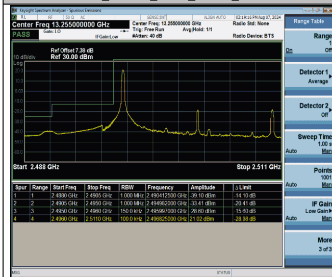
Band41_15MHz_QPSK_39725_1RB#0
