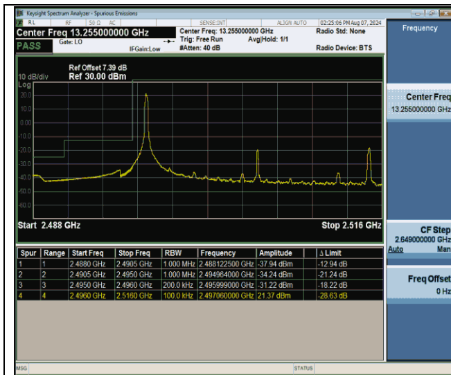
Band41_20MHz_QPSK_39750_1RB#0
