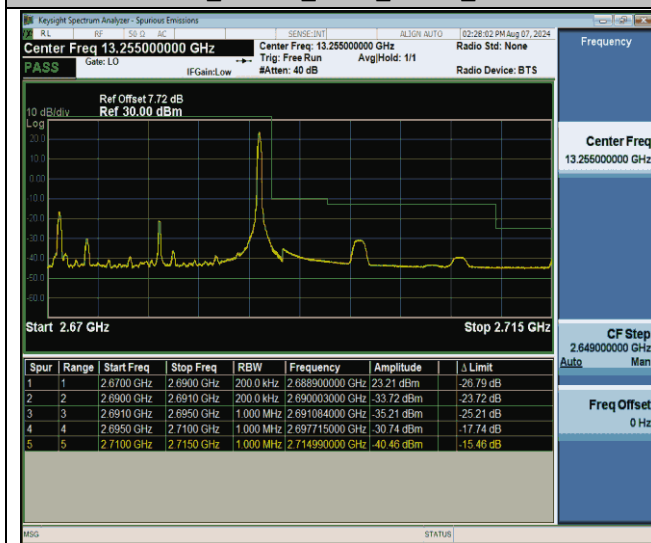
Band41_20MHz_QPSK_41490_1RB#99
