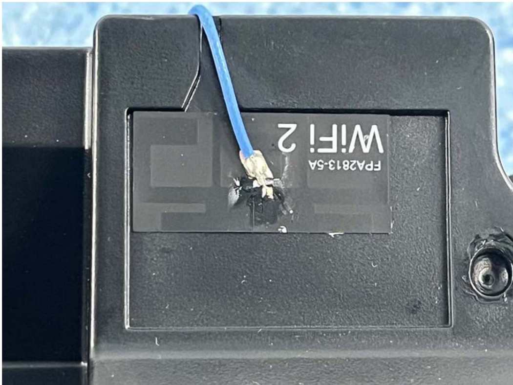
Antenna chain1
