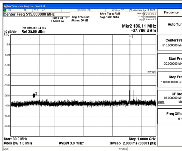
Band5-3MHz-QPSK-20415-1-0-Low-30-1000--37.79-PASS
