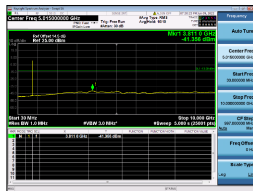
B25-1.4M-High CH-CSE-1-Q16-1 RB 0
