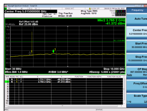
B25-1.4M-High CH-CSE-2-Q16-1 RB 0
