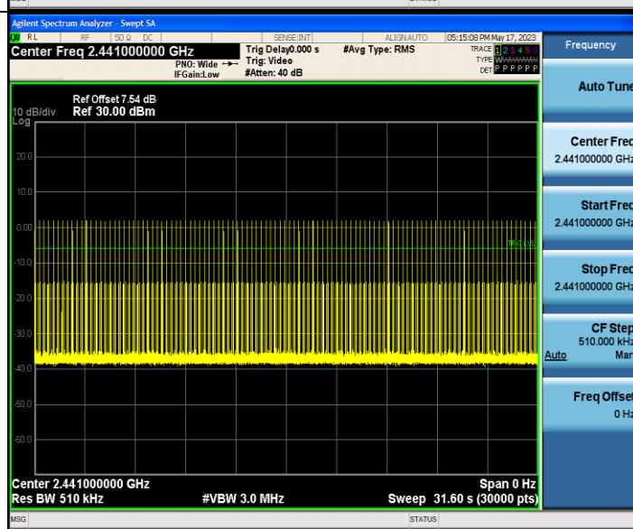
3DH1_Ant1_Hop
