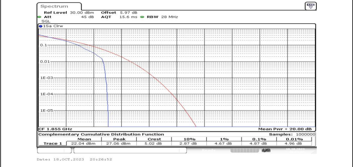
Band2-10MHz-QPSK-18650-1RB#0-PASS
