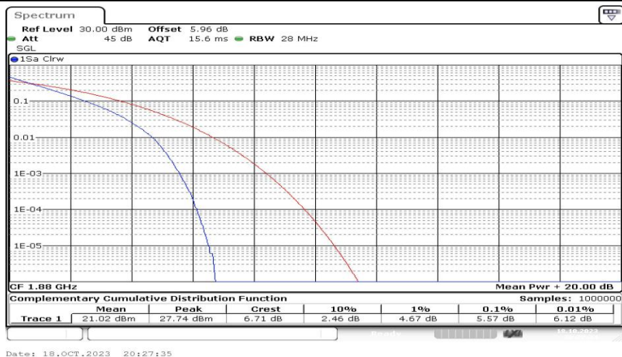
Band2-10MHz-QPSK-18900-50RB#0-PASS
