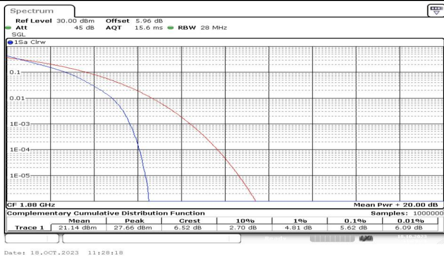
Band2-3MHz-QPSK-18900-15RB#0-PASS
