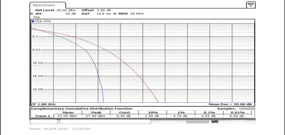
Band2-5MHz-QPSK-18900-25RB#0-PASS
