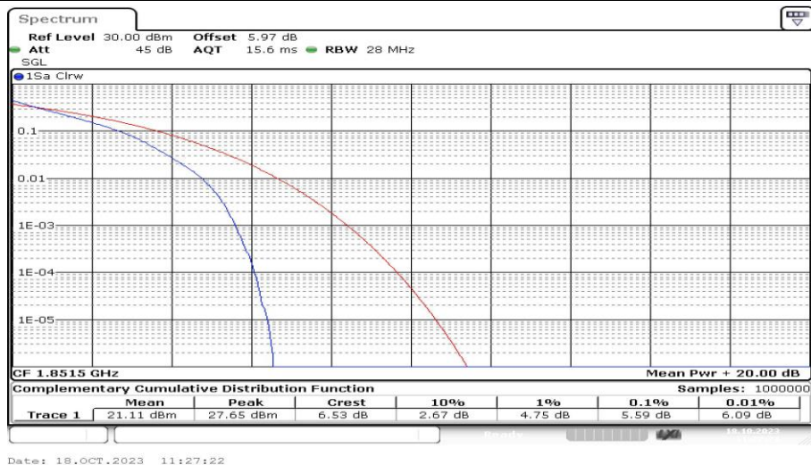
Band2-3MHz-QPSK-18615-15RB#0-PASS
