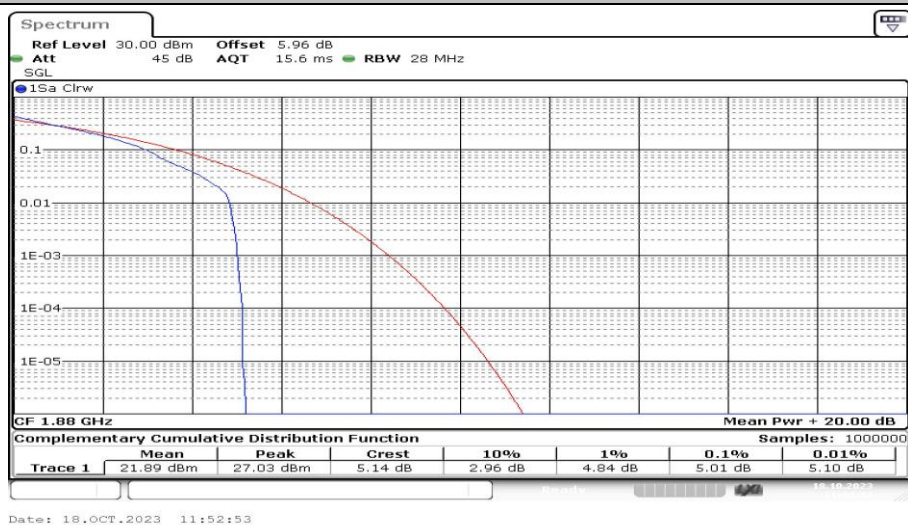
Band2-5MHz-QPSK-18900-1RB#0-PASS
