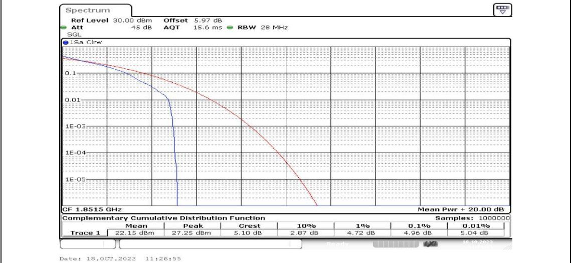
Band2-3MHz-QPSK-18615-1RB#0-PASS
