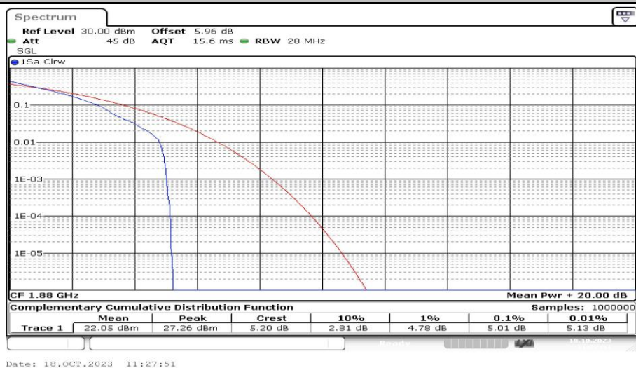
Band2-3MHz-QPSK-18900-1RB#0-PASS
