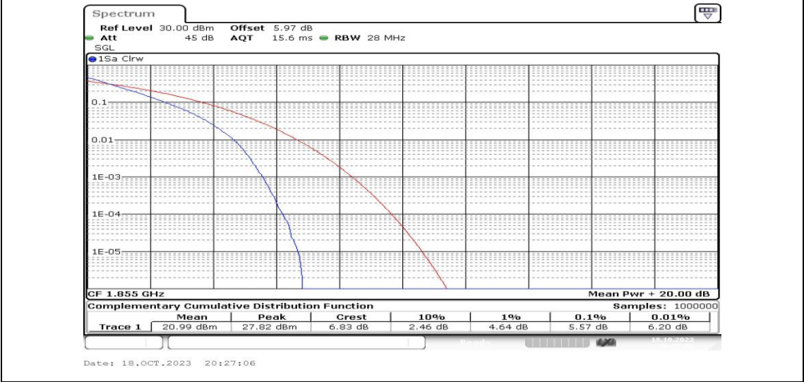
Band2-10MHz-QPSK-18650-50RB#0-PASS
