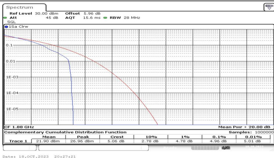
Band2-10MHz-QPSK-18900-1RB#0-PASS
