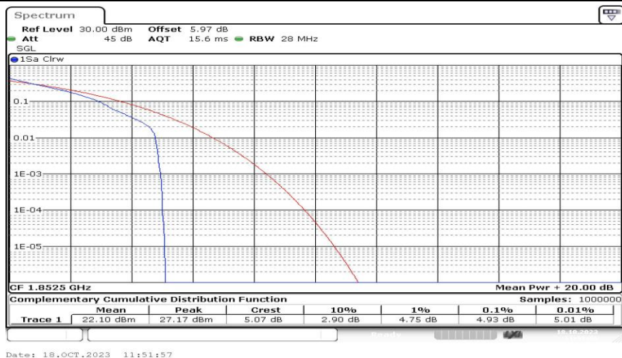
Band2-5MHz-QPSK-18625-1RB#0-PASS
