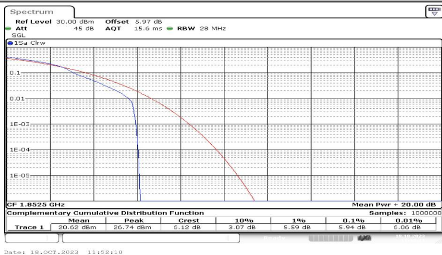
Band2-5MHz-16QAM-18625-1RB#0-PASS
