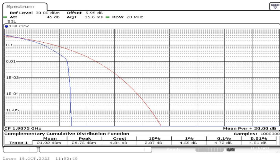
Band2-5MHz-QPSK-19175-1RB#0-PASS
