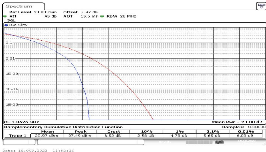
Band2-5MHz-QPSK-18625-25RB#0-PASS
