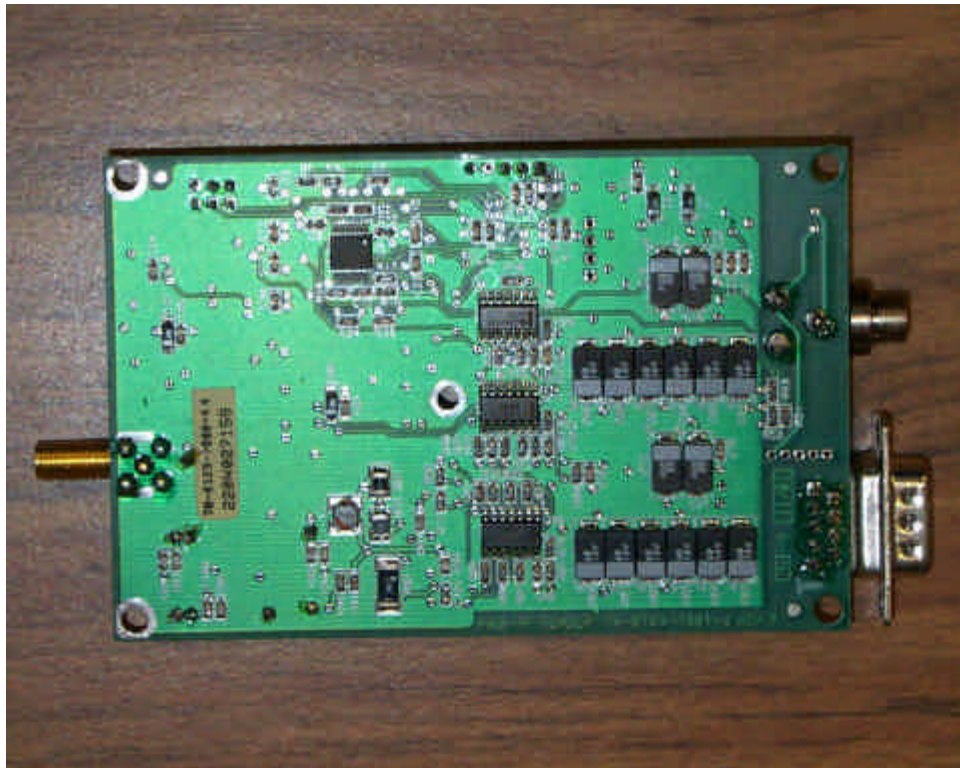
3M Reader PCB Bottom
