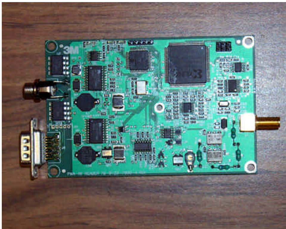
3M Reader PCB Top
