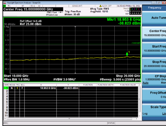
B4-5M-High CH-PAPR-Q16
