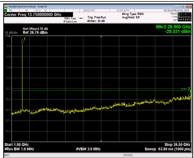
Band7-20MHz-64QAM-21350-1RB#0-Range2:1000~265 00MHz
