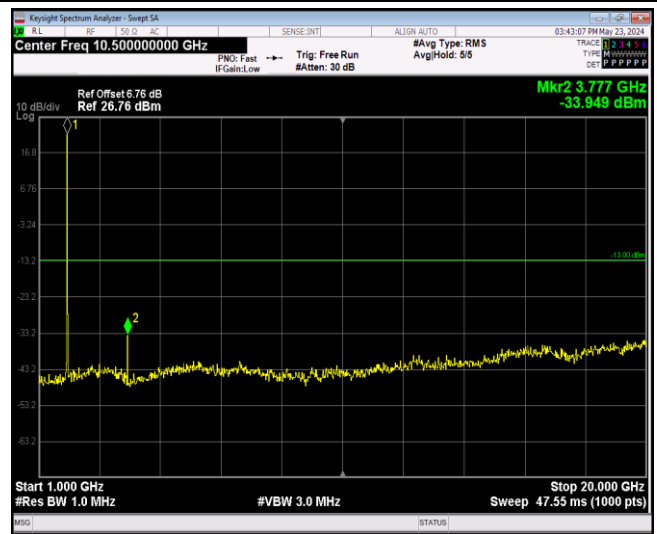
Band2-20MHz-16QAM-19100-1RB#0-Range2:1000~200 00MHz
