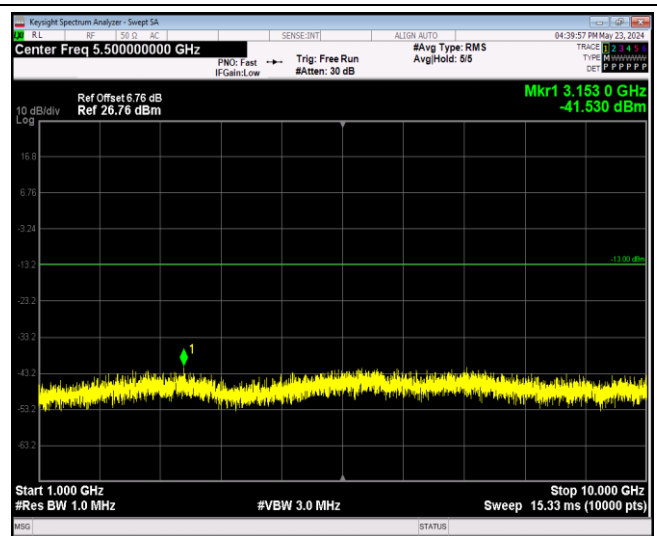
Band5-10MHz-QPSK-20525-1RB#0-Range2:1000~1000 OMHz
