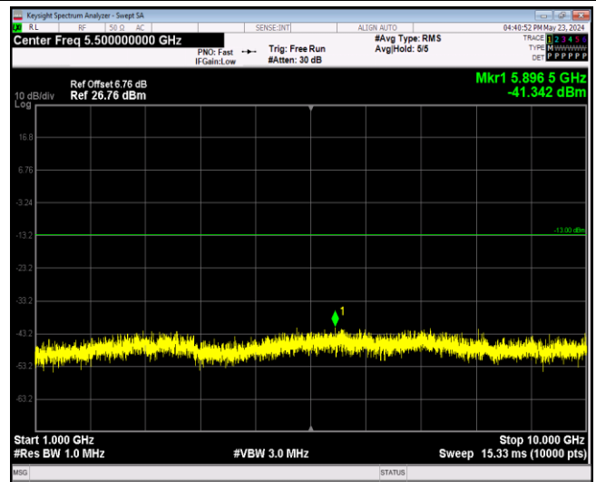
Band5-10MHz-QPSK-20600-1RB#0-Range2:1000~1000 OMHz
