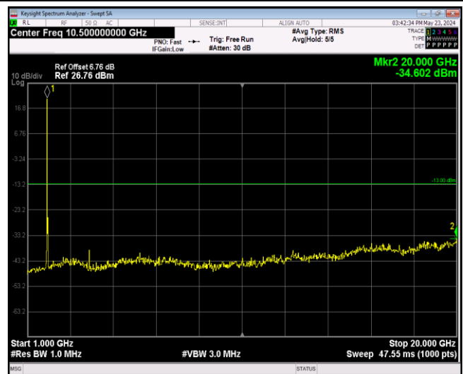
Band2-20MHz-64QAM-19100-1RB#0-Range2:1000~200 00MHz
