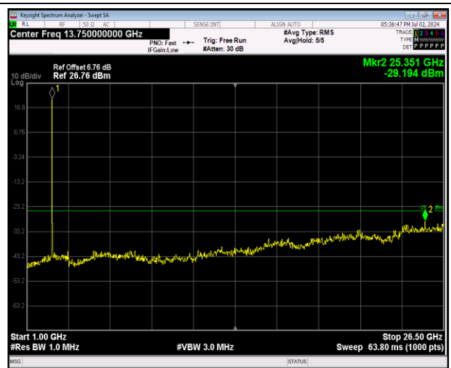
Band7-20MHz-16QAM-20850-1RB#0-Range2:1000~265 00MHz
