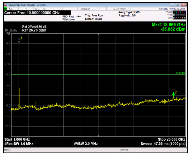
Band2-20MHz-64QAM-18900-1RB#0-Range2:1000~200 00MHz
