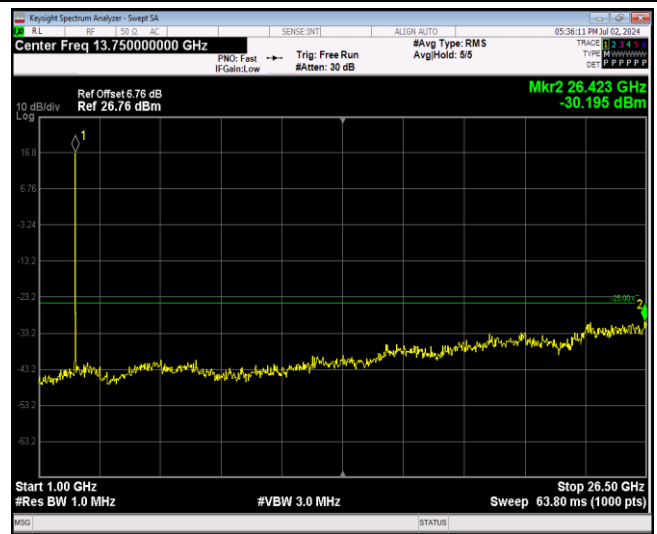
Band7-20MHz-16QAM-21100-1RB#0-Range2:1000~265 00MHz
