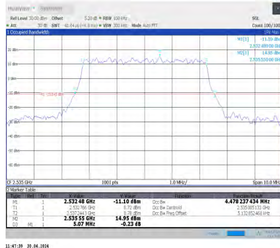
1-N7-PC3-15-5-M-4-DFT-64QAM-Outet_Full-25@0-A Ant0-4.478-5.070-≤5-PASS
