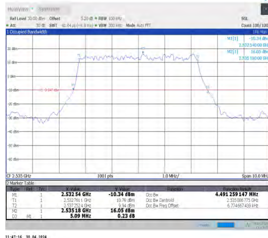
1-N7-PC3-15-5-M-2-DFT-PI2BPSK-Outet_Full-25@0-A Ant0-4.491-5.090-≤5-PASS
