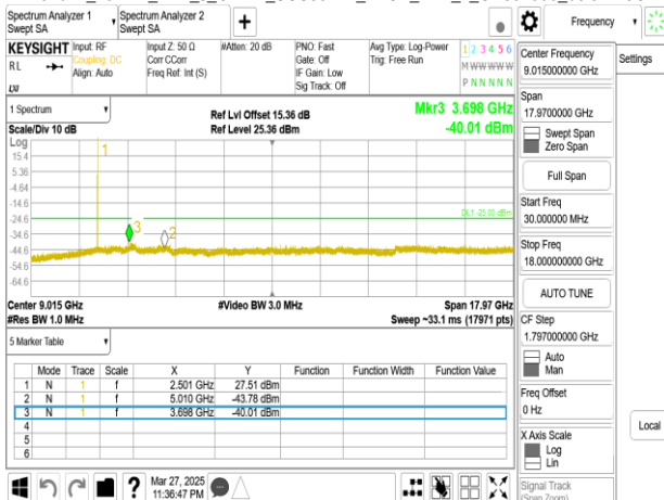
Band41_10MHz_DFT_s_OFDM_SCS30kHz_BPSK_RB1_1_CH501000upper 18G
