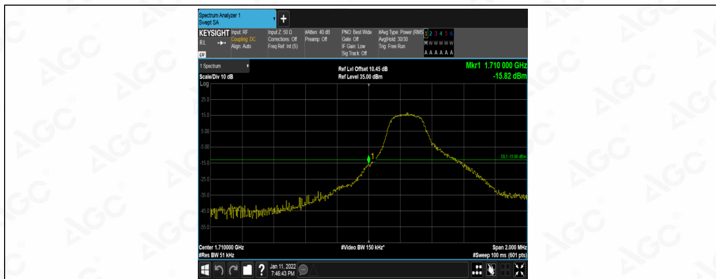
Band4-3MHz-QPSK-19965-1RB#14
