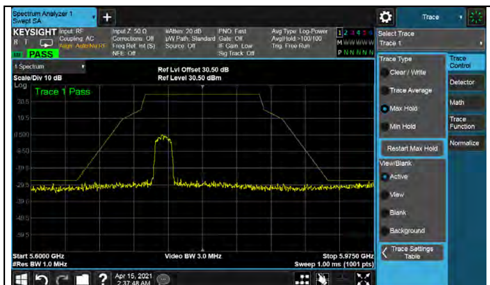
802.11n(HT20)-5745MHz
