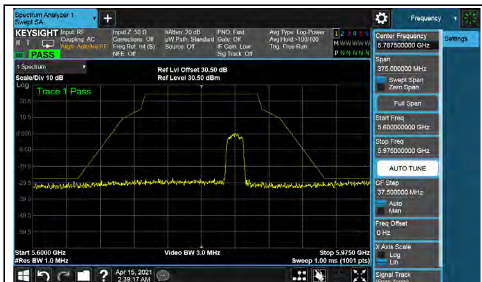
802.11n(HT20)-5825MHz
