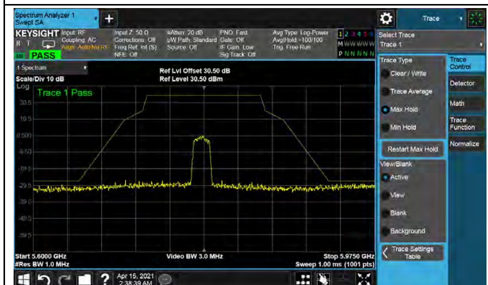
802.11n(HT20)-5785MHz
