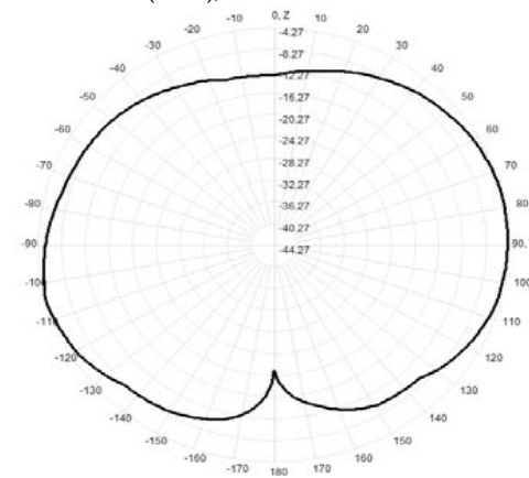
916.0MHz Total(E2-YZ), Max= -4.27dBi
