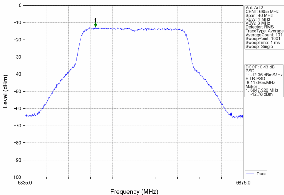
802.11ax(HEW20)_HCH_6855MHz_RU242_Left_Ant2_NTNV
