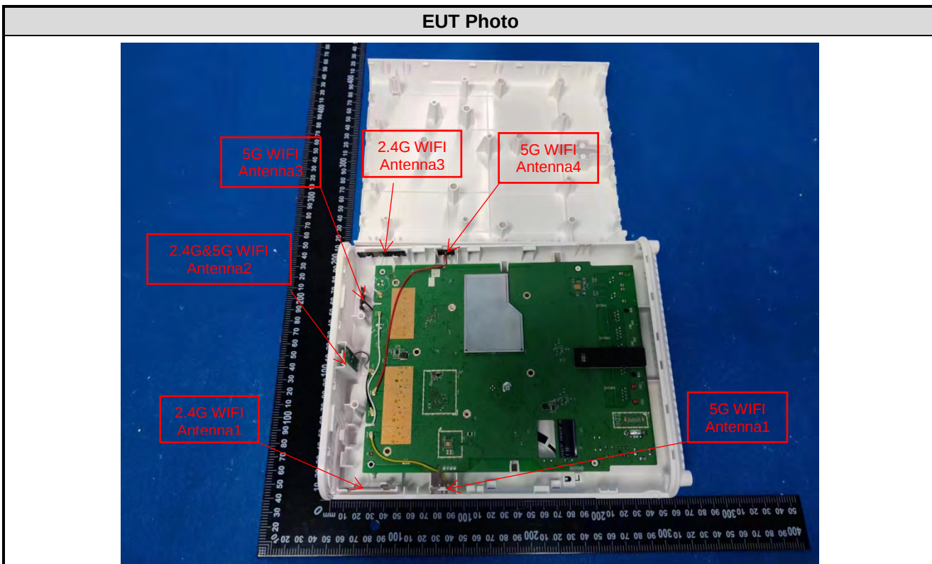
EUT Photo
