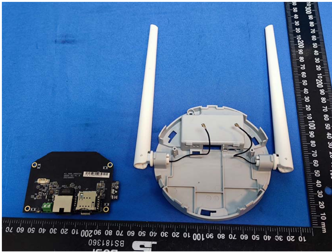
4G Antenna
