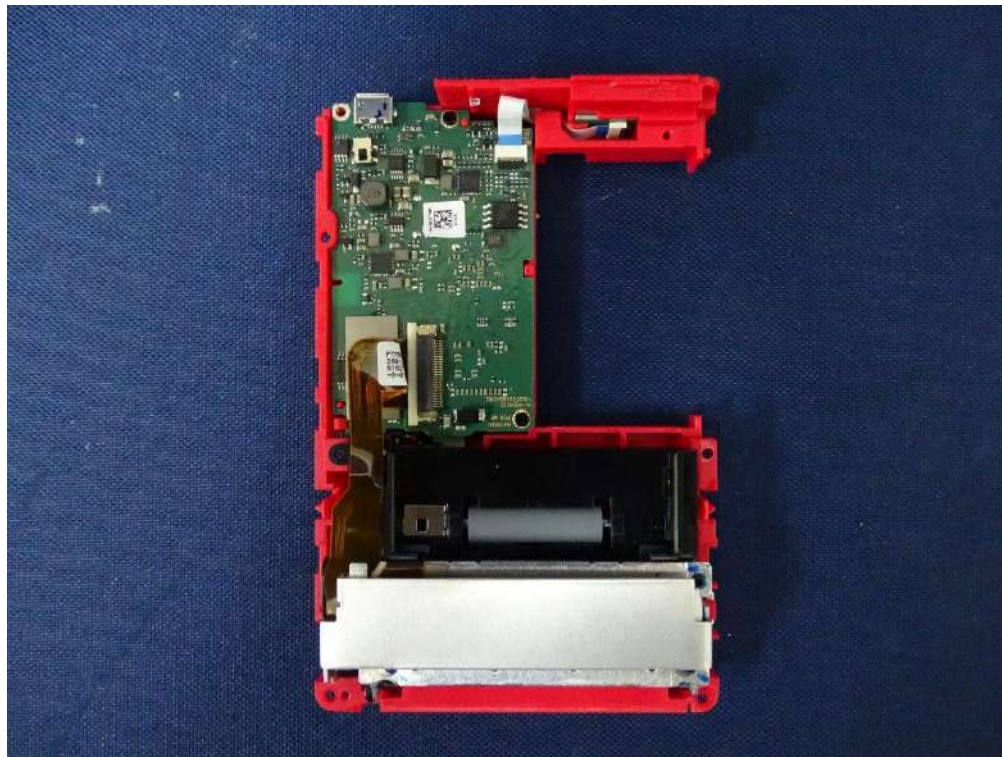
(19) EUT Photo
