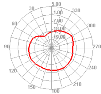
2690.000MHz H
