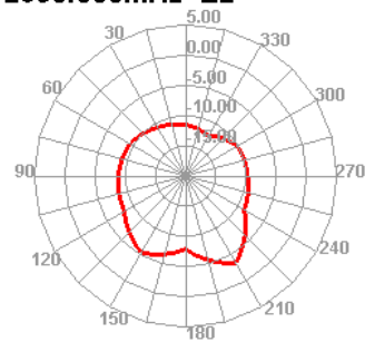
2690.000MHz E2
