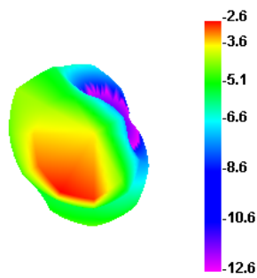
1990.000MHz E1
