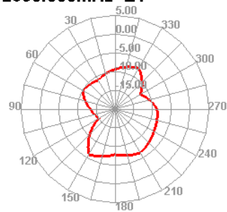
2690.000MHz E1
