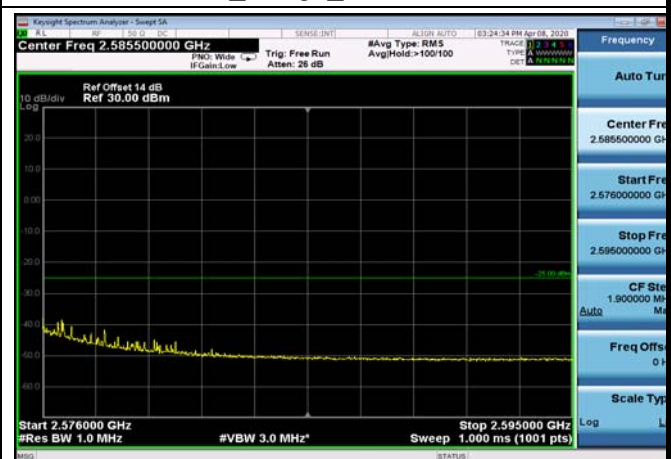
FDD07_5MHz_2567.5_QPSK_fullIRB_ExtraBa nds_Range_2576~2595
