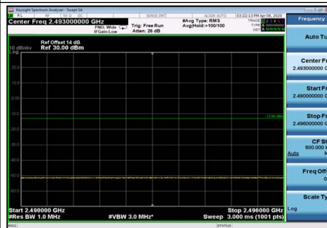
FDD07_5MHz_2567.5_QPSK_OneRB_low _ExtraBands_Range_2490~2496
