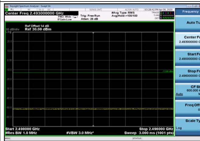
FDD07_10MHz_2565_QPSK_fullIRB_ExtraBan ds_Range_2490~2496
