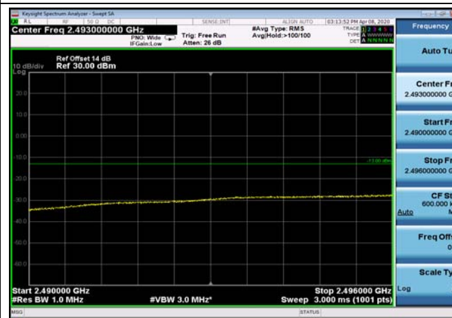
FDD07_15MHz_2507.5_Q16_fullIRB_ExtraBa nds_Range_2490~2496
