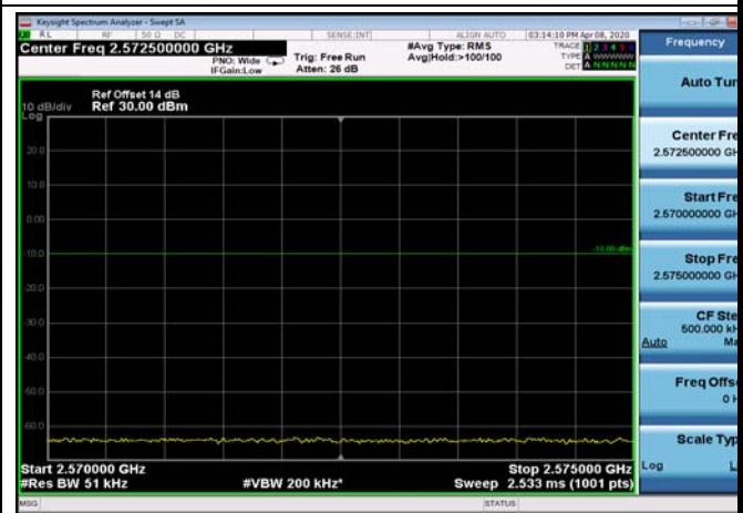
FDD07_15MHz_2507.5_Q16_fullIRB_ExtraBa nds_Range_2570~2575
