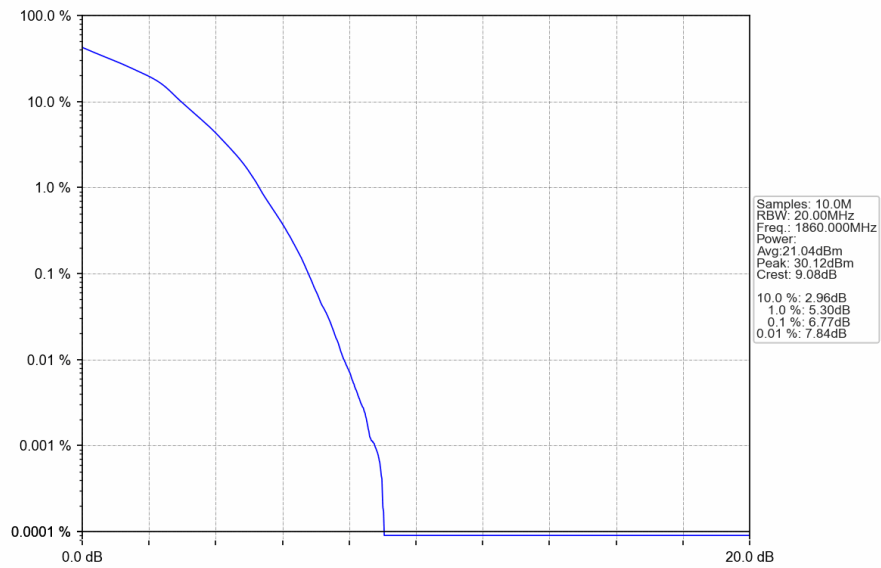
Band2_20MHz_16QAM_LCH_1860MHz_RB_27_0_NTNV
