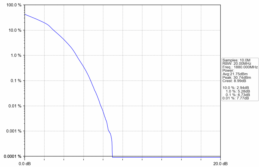
Band2_20MHz_16QAM_MCH_1880MHz_RB_27_0_NTNV
