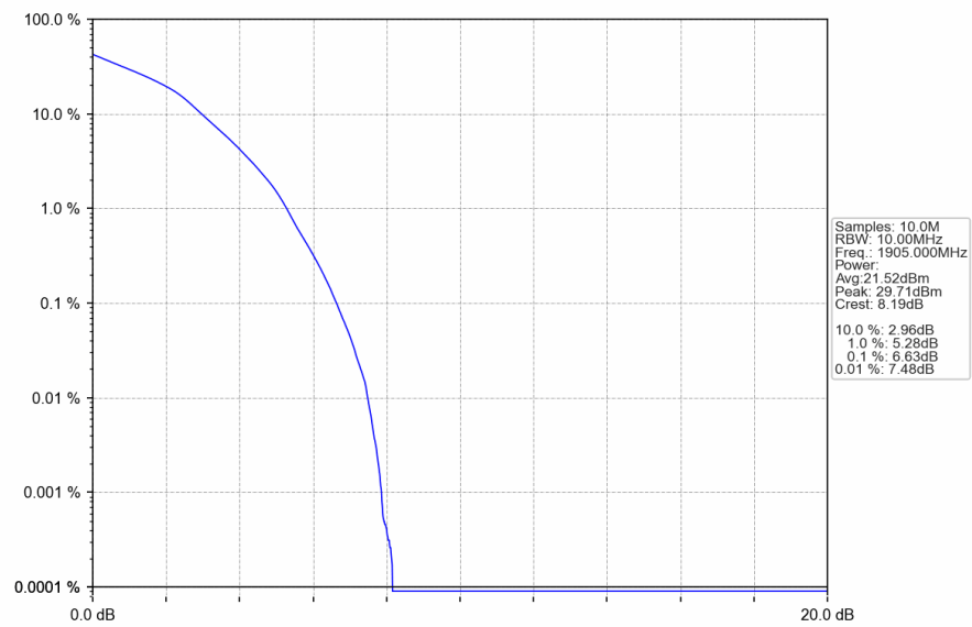
Band2_10MHz_16QAM_HCH_1905MHz_RB_27_23_NTNV
