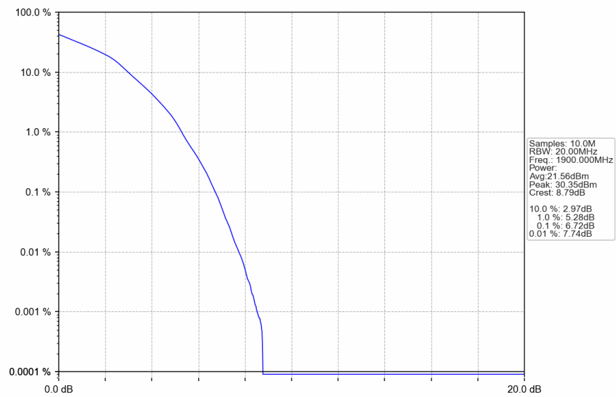
Band2_20MHz_16QAM_HCH_1900MHz_RB_27_73_NTNV
