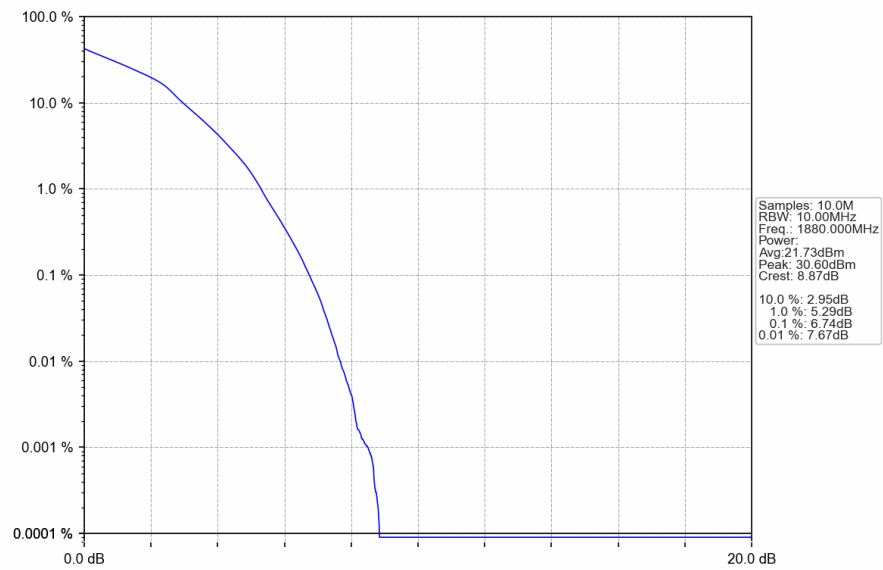
Band2_10MHz_16QAM_MCH_1880MHz_RB_27_0_NTNV
